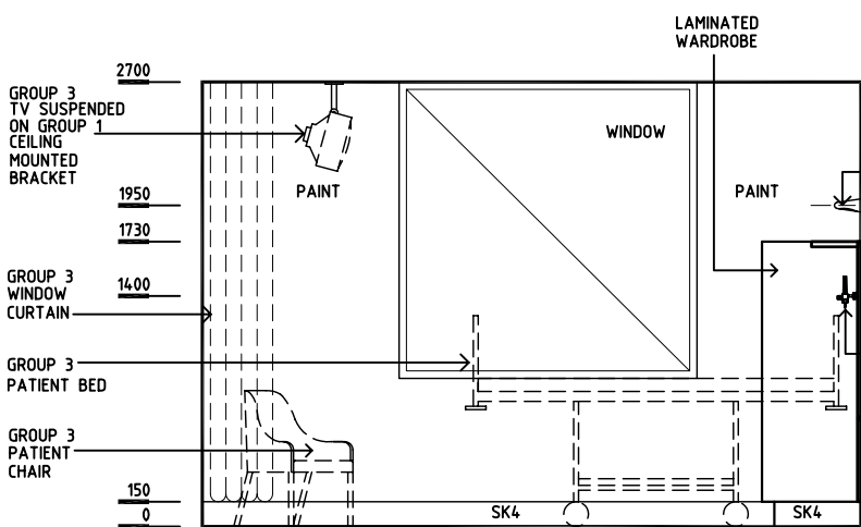
ELEVATION 1
