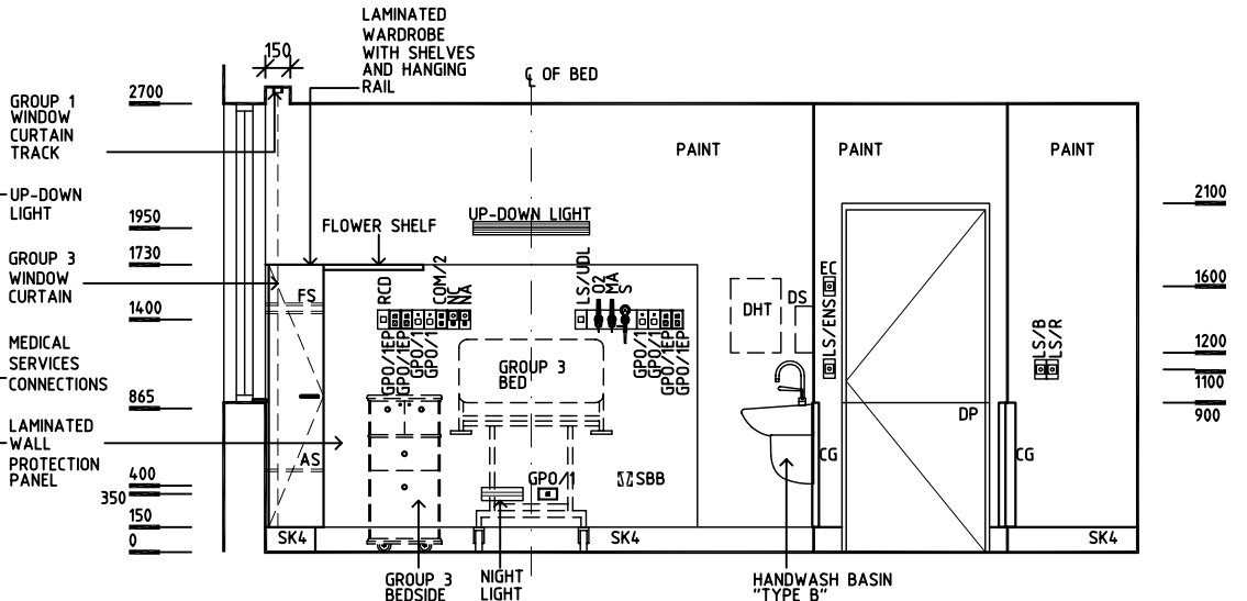
ELEVATION 2
