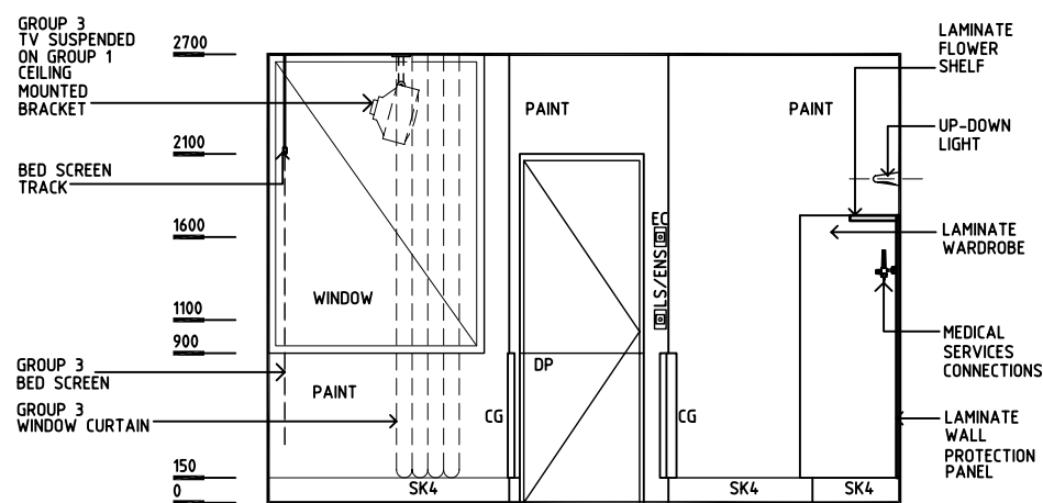
ELEVATION 1
