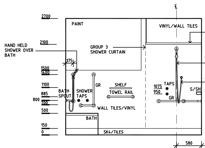
ELEVATION 1
