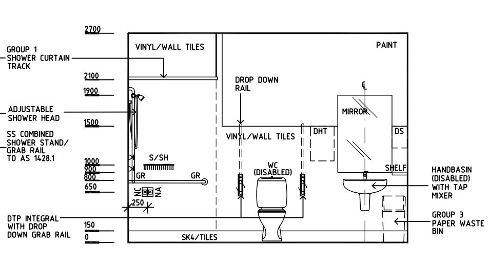
ELEVATION 2
