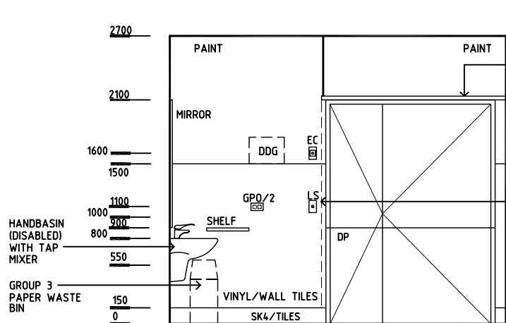
ELEVATION 3
