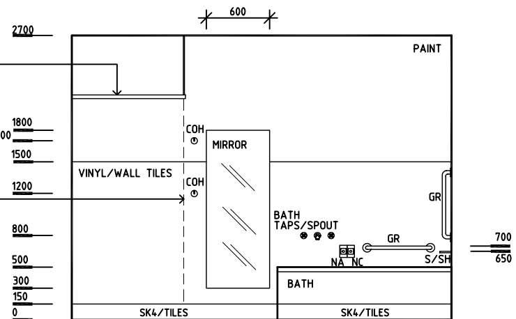
ELEVATION 4
