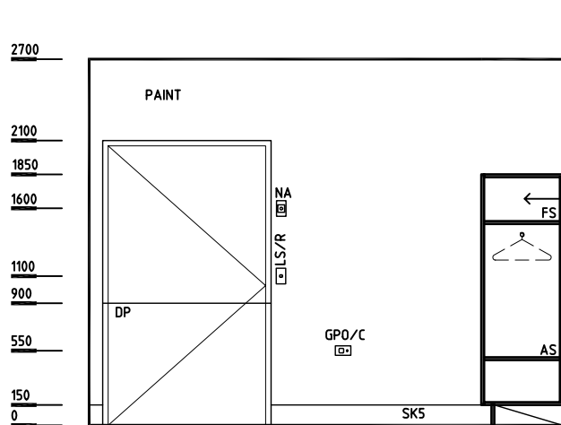
ELEVATION 3
