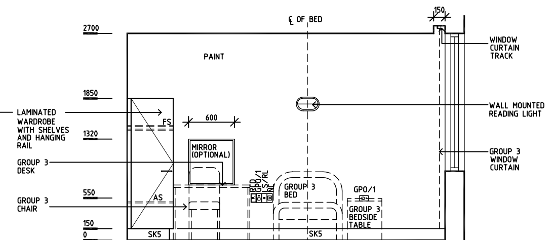
ELEVATION 4
