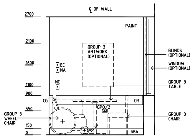
ELEVATION 2
