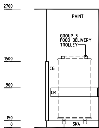
ELEVATION 1
