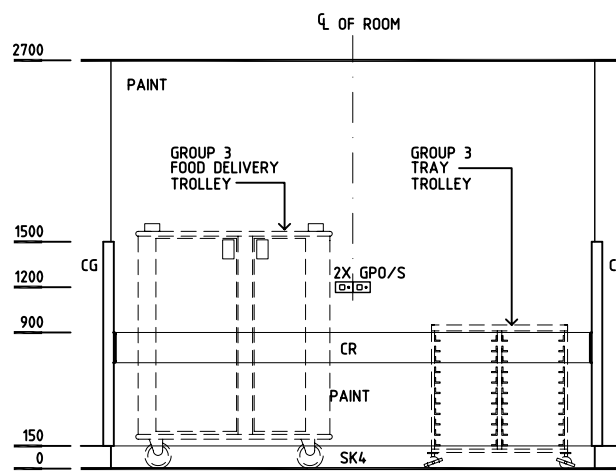
ELEVATION 2
