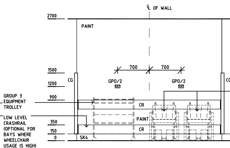
ELEVATION 2
