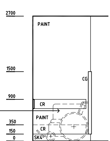
ELEVATION 3
