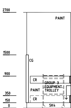
ELEVATION 1
