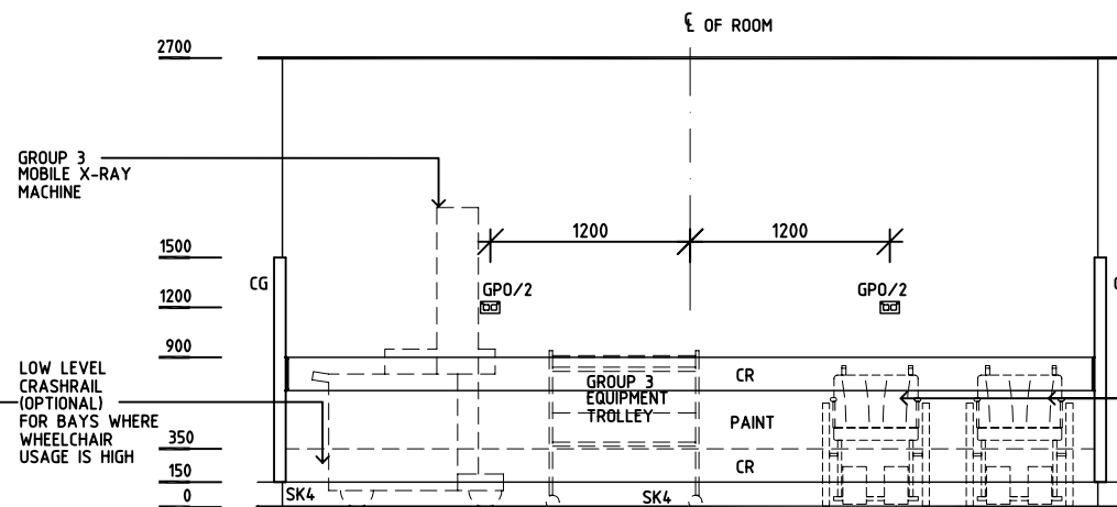
ELEVATION 2
