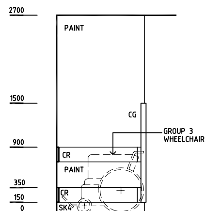
ELEVATION 3
