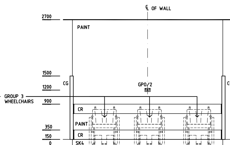
ELEVATION 2
