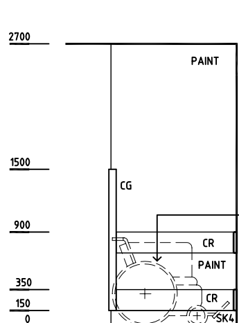
ELEVATION 1
