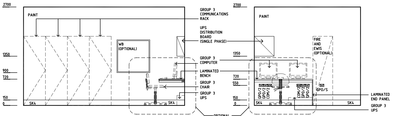
ELEVATION 1
