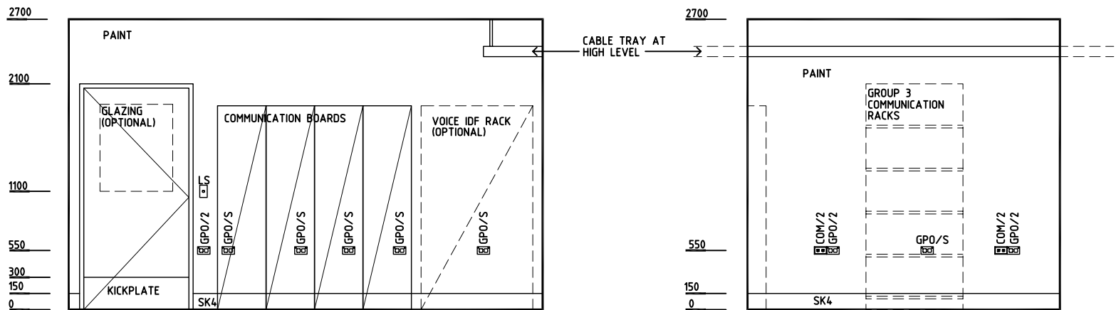
ELEVATION 3
