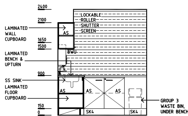
ELEVATION 5
