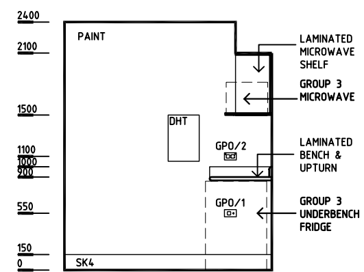
ELEVATION 6
