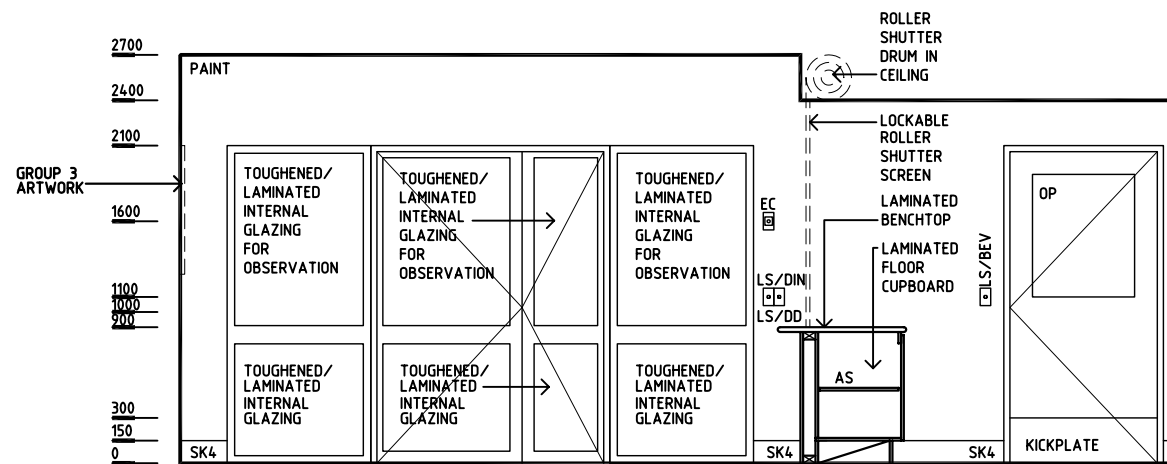
ELEVATION 2
