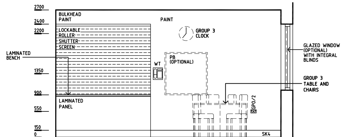
ELEVATION 4
