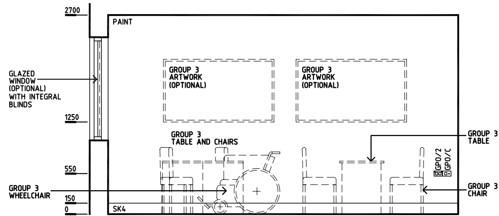
ELEVATION 2
