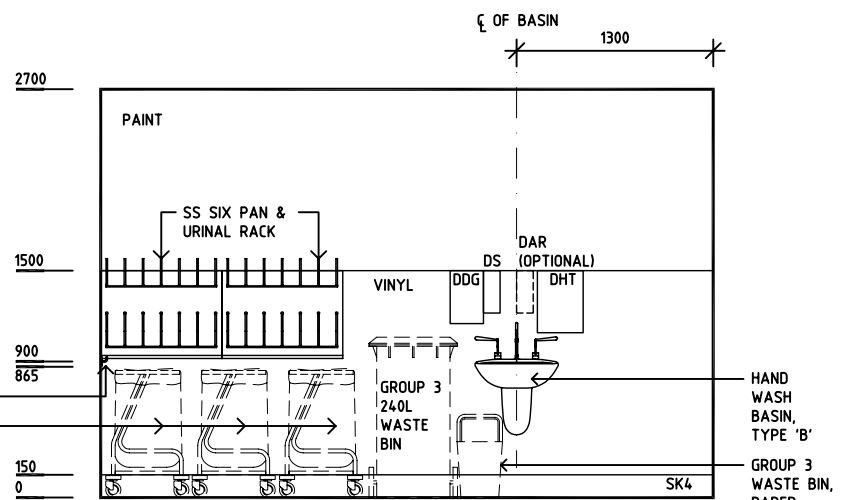
ELEVATION 2
