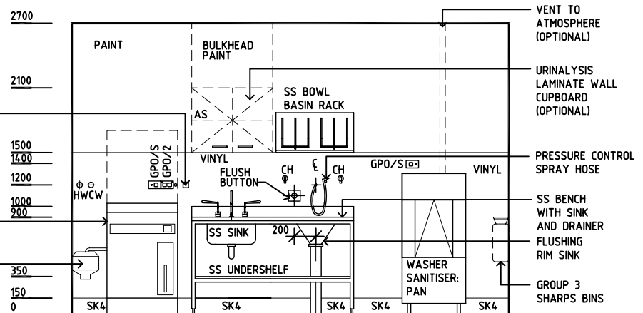
ELEVATION 4
