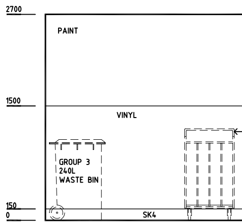
ELEVATION 1
