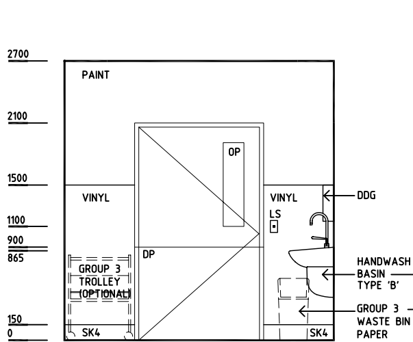
ELEVATION 1
