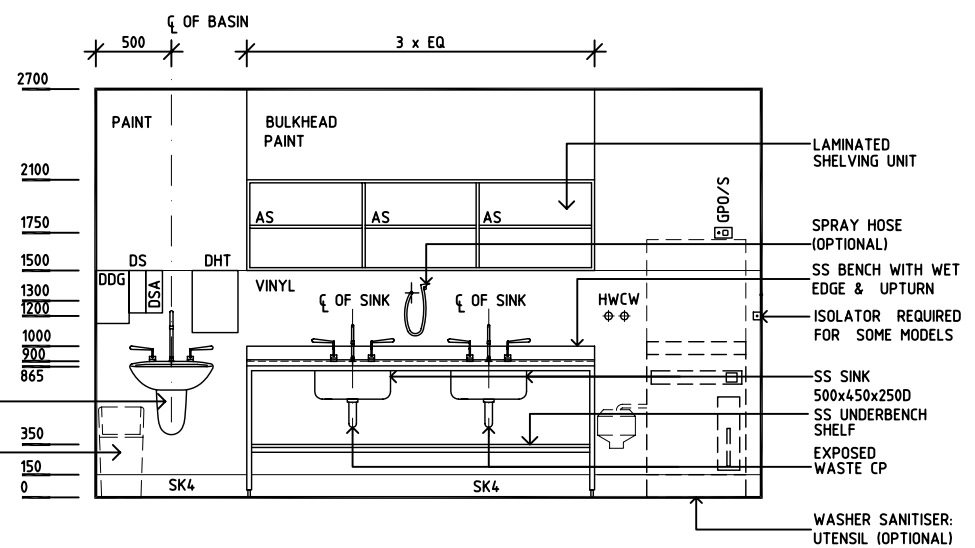
ELEVATION 4
