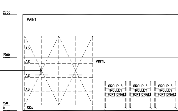
ELEVATION 2
