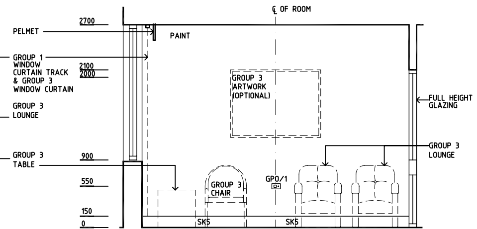
ELEVATION 2
