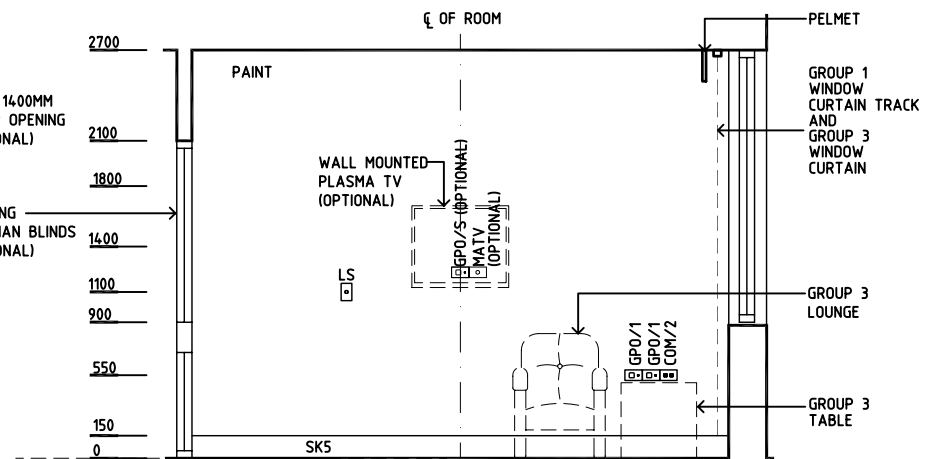
ELEVATION 4
