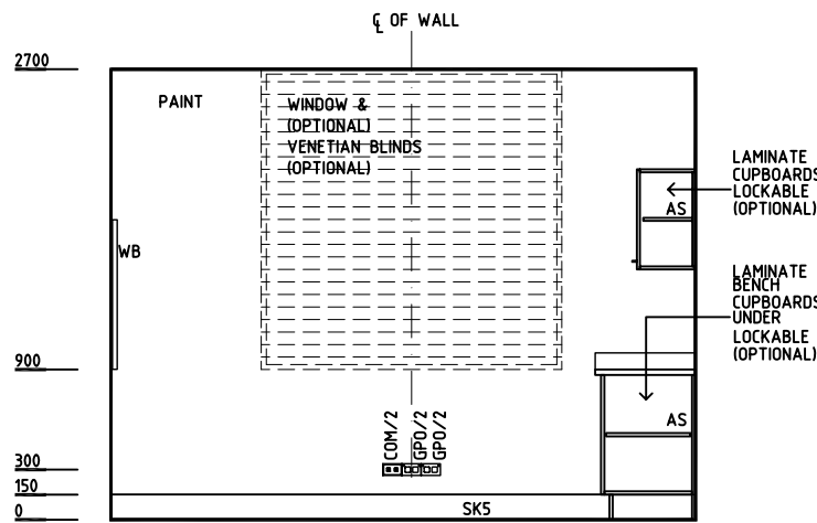
ELEVATION 1
