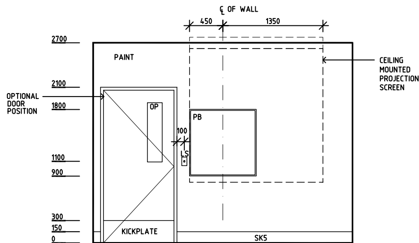
ELEVATION 3
