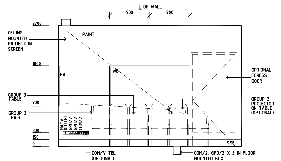
ELEVATION 4
