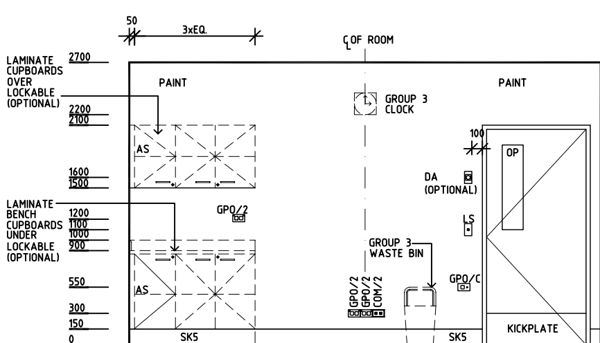
ELEVATION 3
