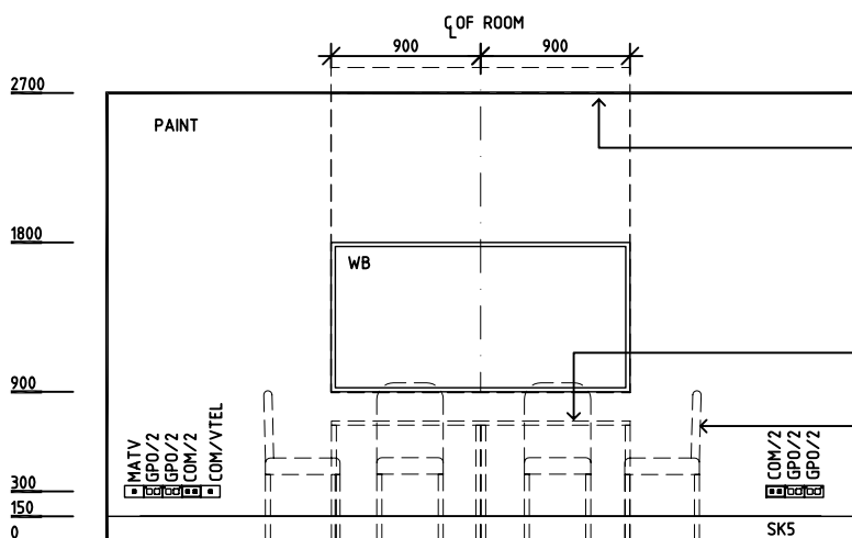
ELEVATION 1
