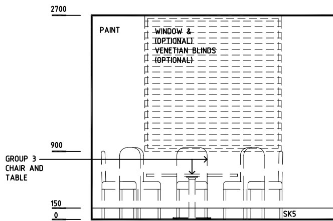
ELEVATION 1
