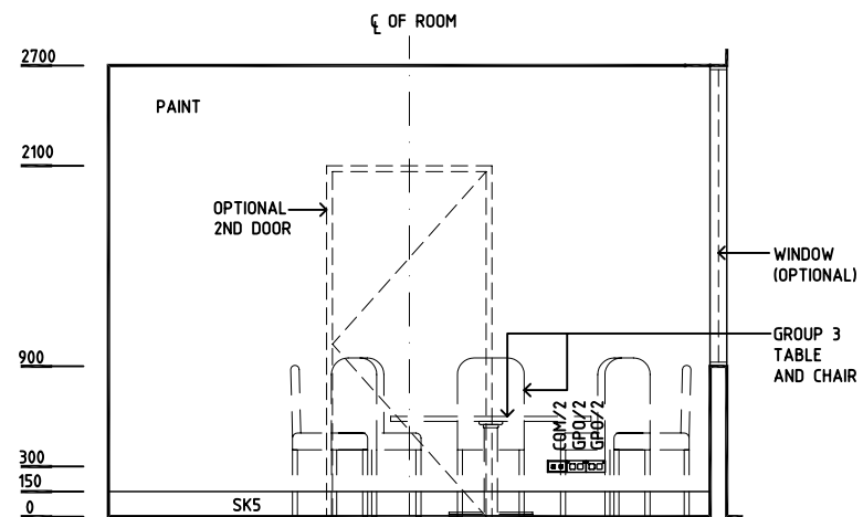
ELEVATION 4
