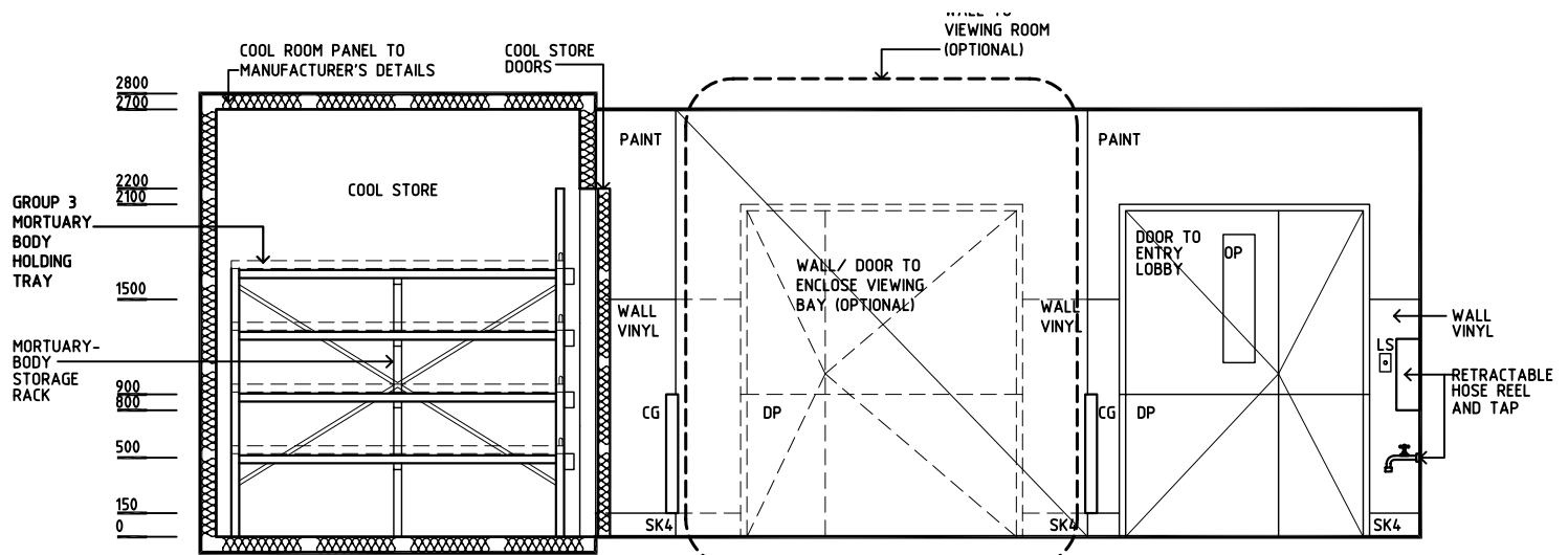
ELEVATION 1
