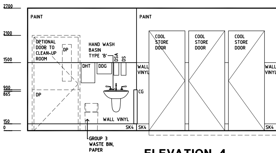
ELEVATION 4
