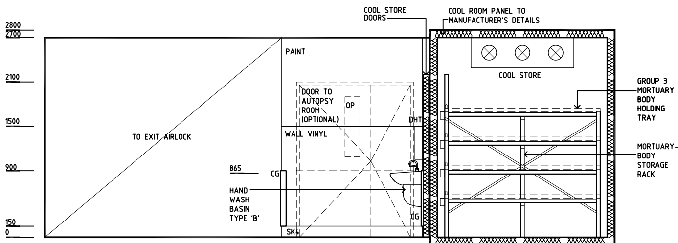
ELEVATION 3
