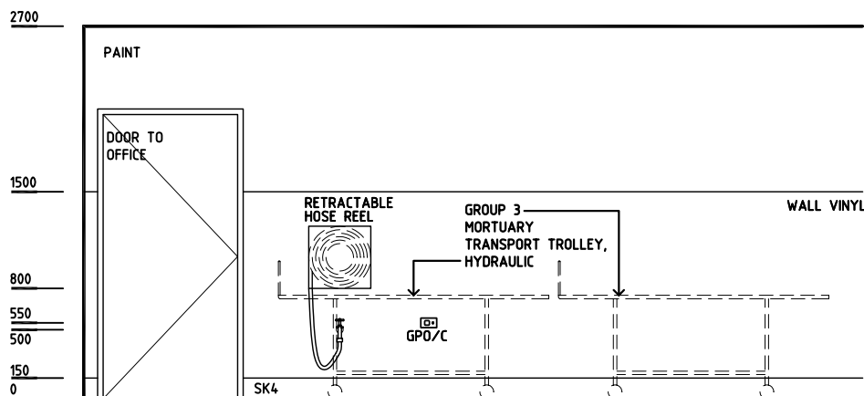
ELEVATION 2
