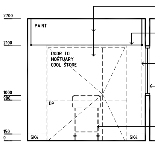
ELEVATION 3
