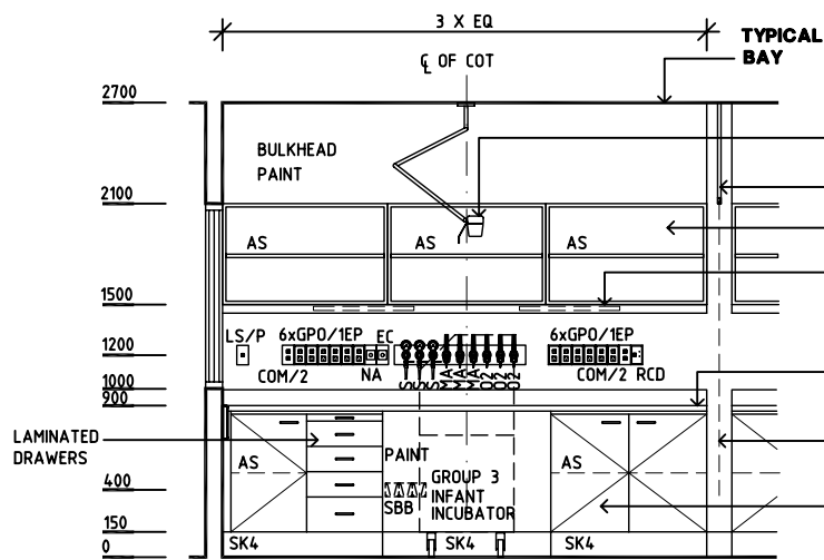
ELEVATION 1
