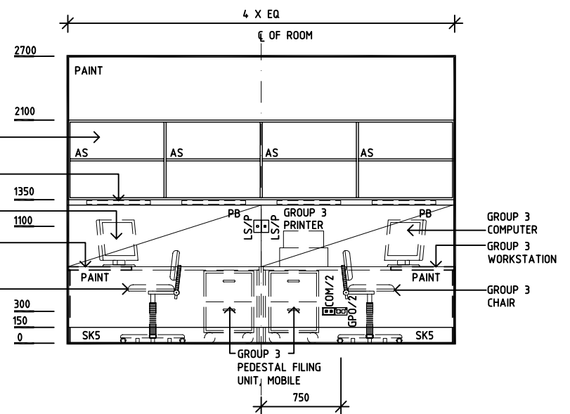
ELEVATION 2
