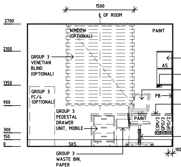
ELEVATION 1
