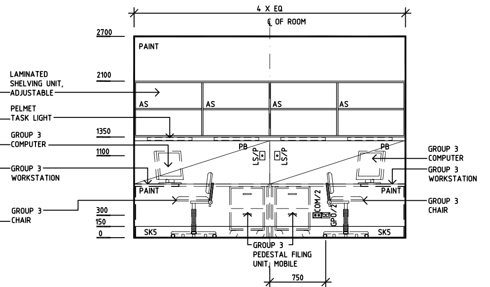
ELEVATION 2
