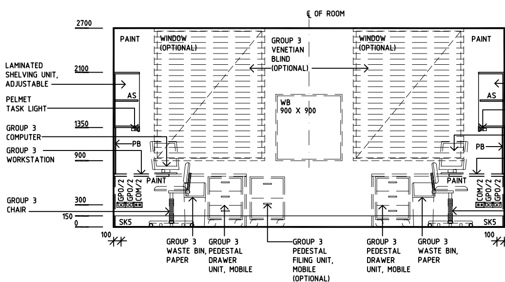
ELEVATION 1
