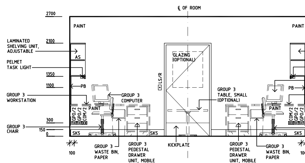
ELEVATION 3
