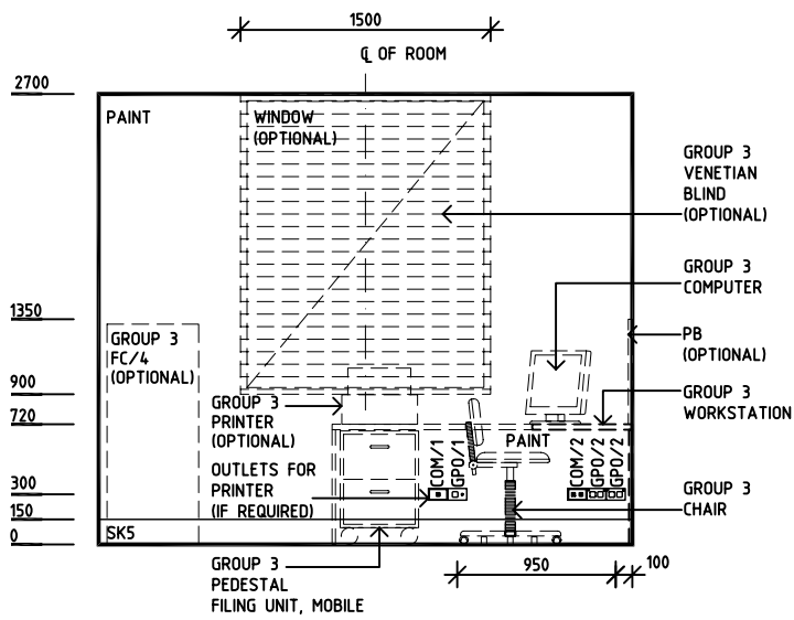
ELEVATION 1
