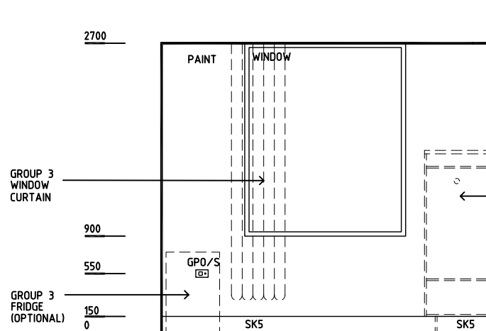
ELEVATION 1
