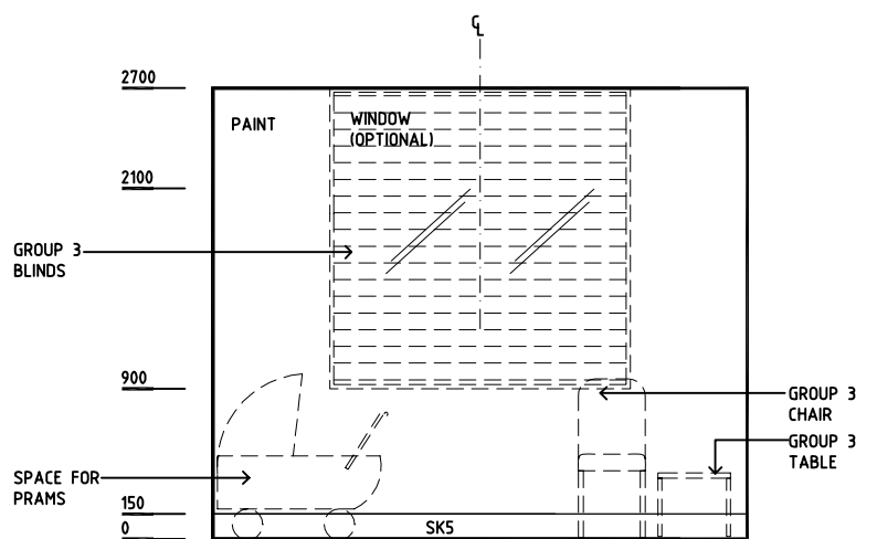
ELEVATION 1
