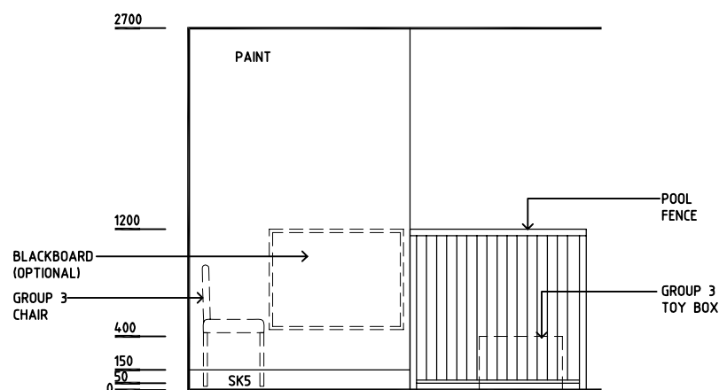
ELEVATION 2
