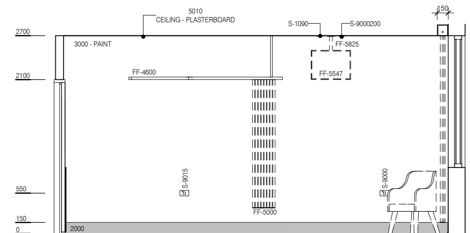
ELEVATION 4
