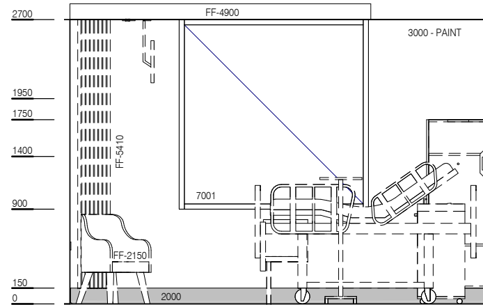
ELEVATION 1
