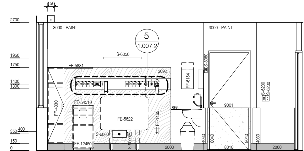
ELEVATION 2
