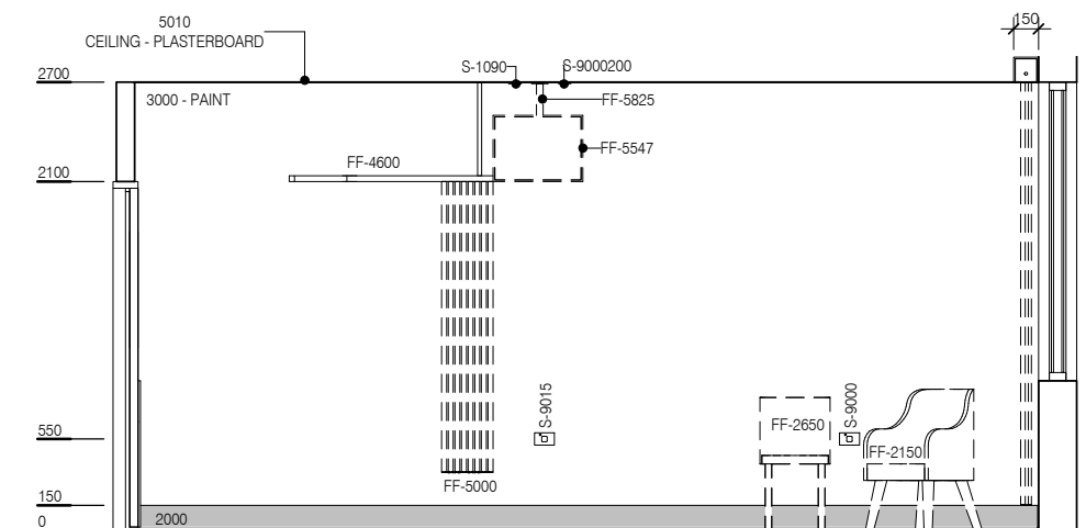
ELEVATION 4
