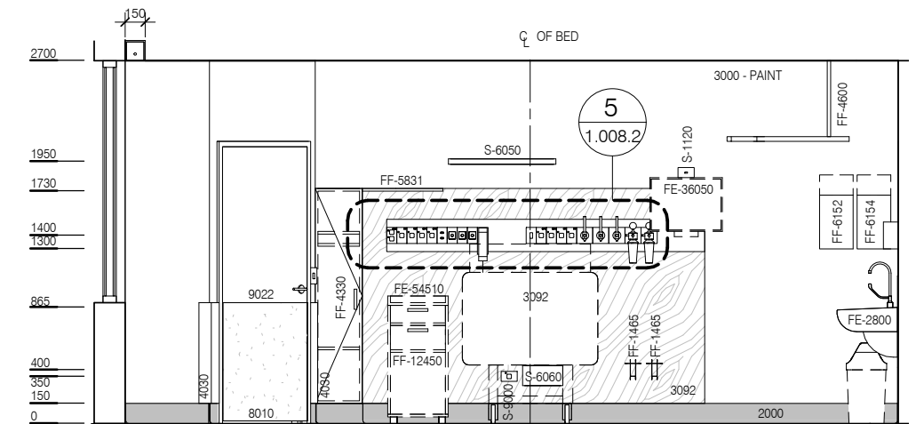
ELEVATION 2
