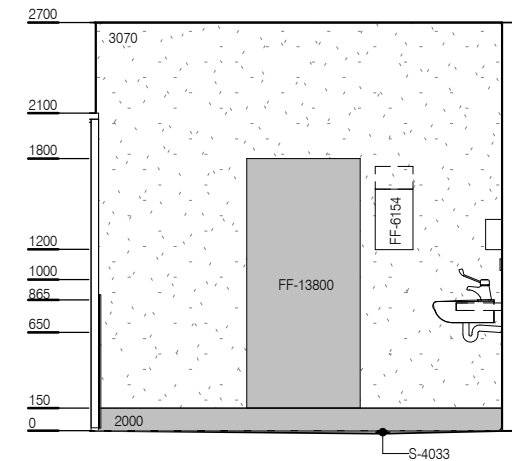
ELEVATION 4
