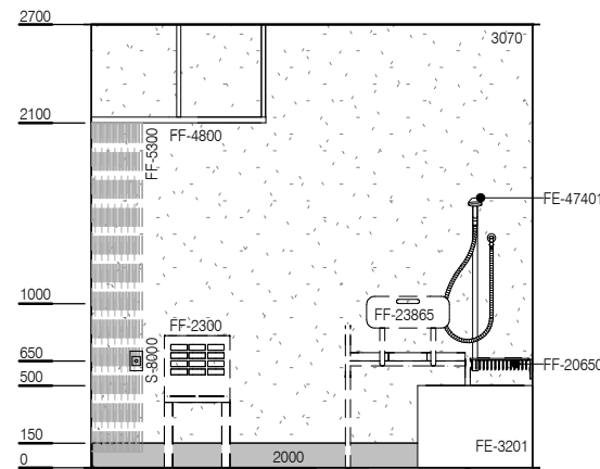
ELEVATION 2
