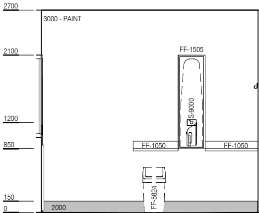
ELEVATION 4
