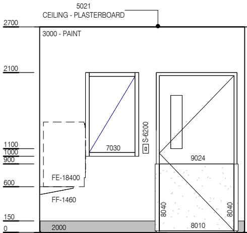
ELEVATION 3
