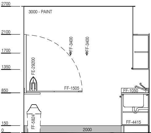
ELEVATION 1
