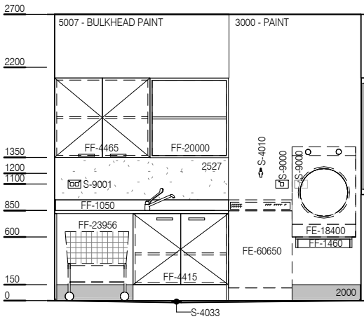
ELEVATION 2
