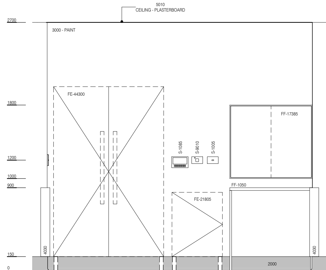
ELEVATION 2
