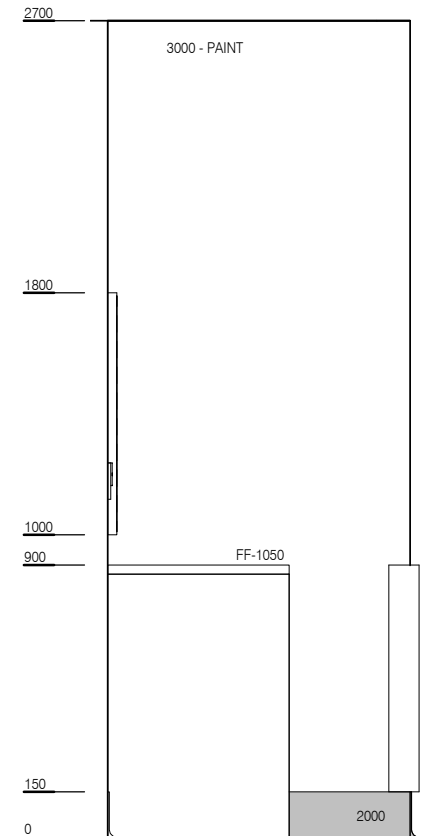
ELEVATION 3
