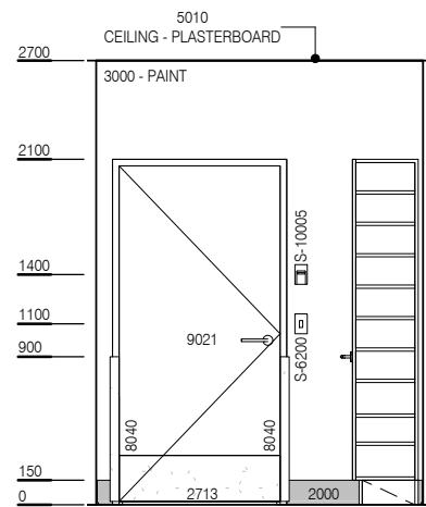
ELEVATION 2
