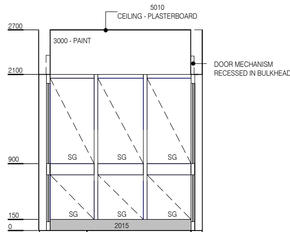
ELEVATION 2
