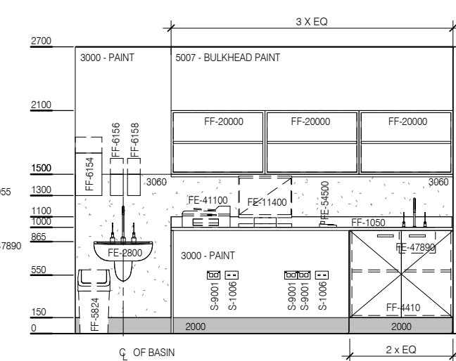
ELEVATION 4
