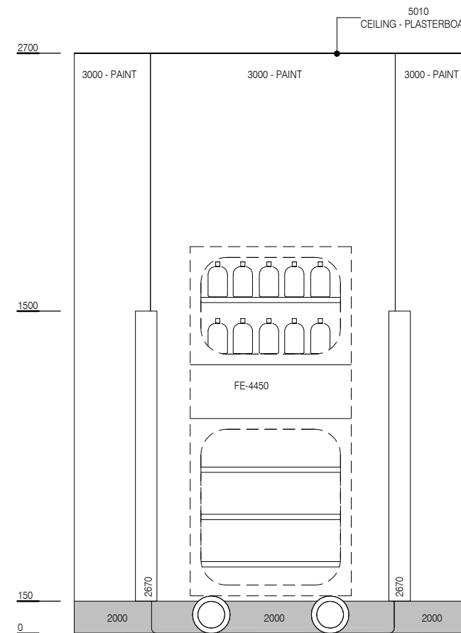
ELEVATION 2
