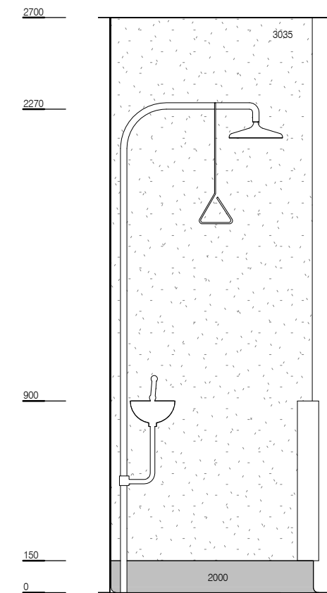
ELEVATION 2
