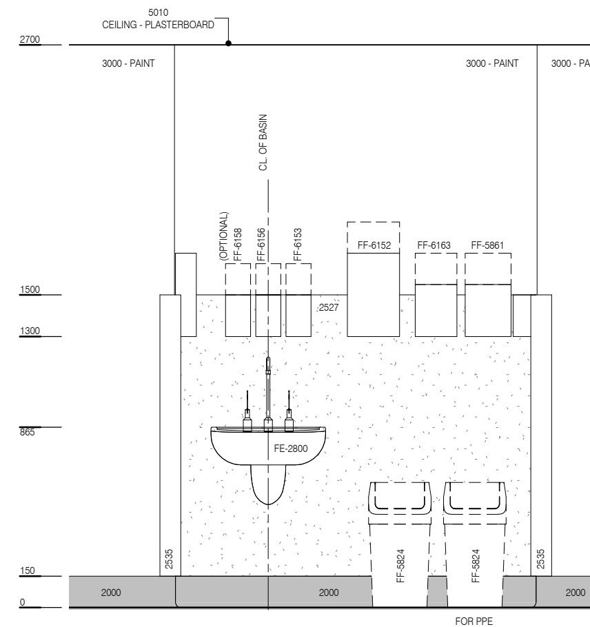
ELEVATION 2
