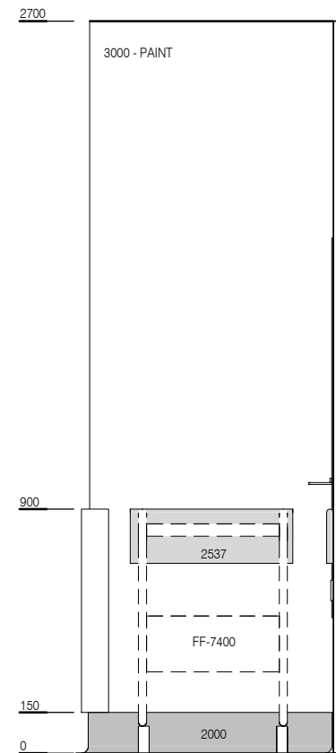
ELEVATION 1
