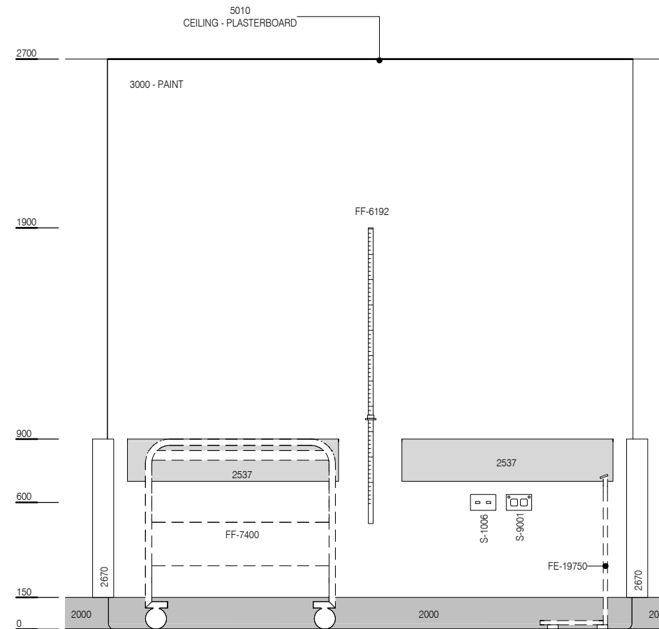
ELEVATION 2
