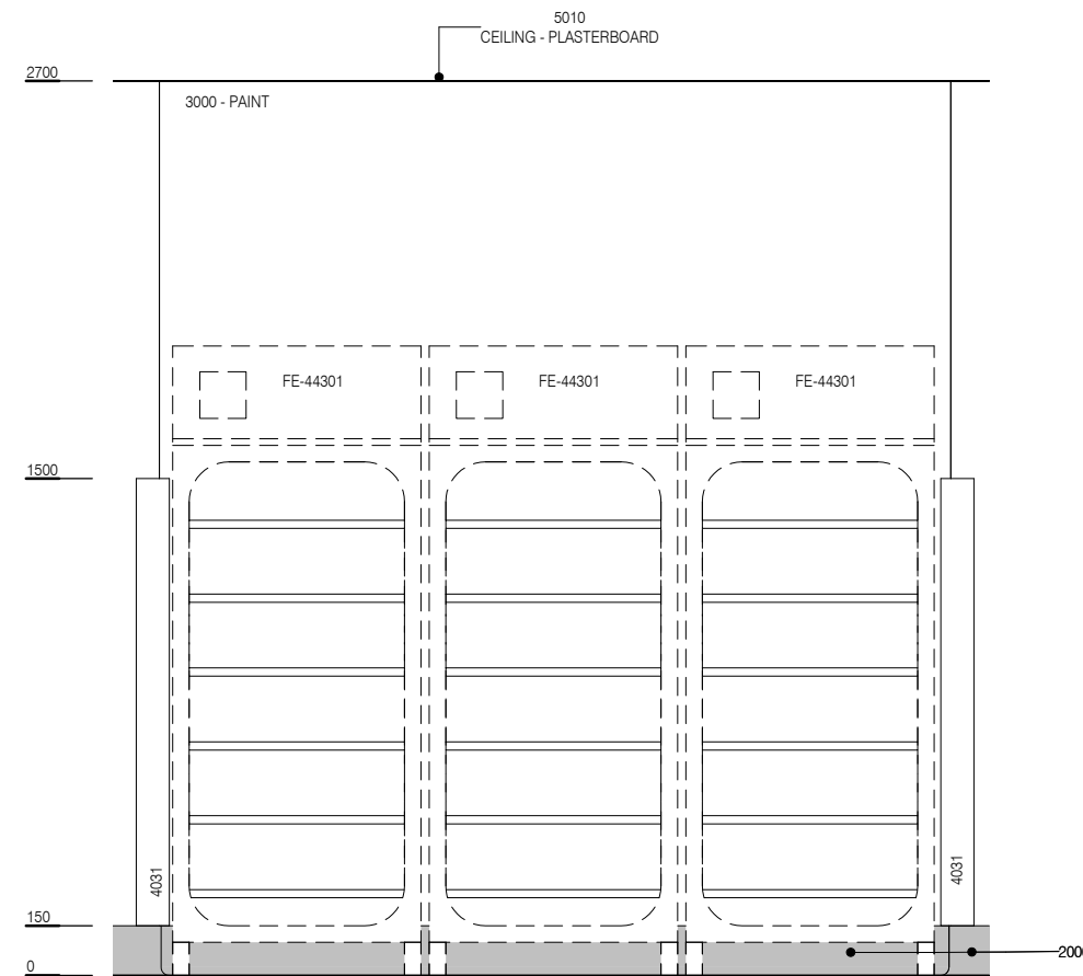
ELEVATION 2
