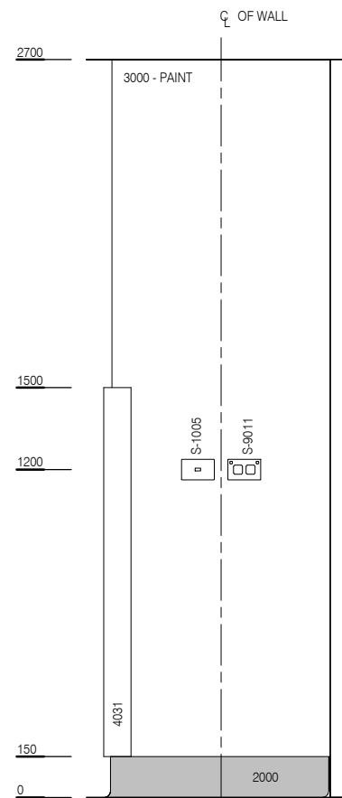
ELEVATION 1
