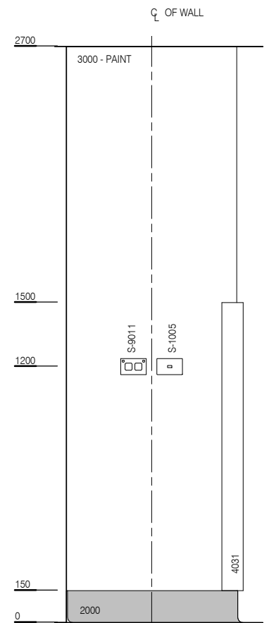
ELEVATION 3
