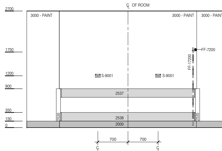
ELEVATION 2
