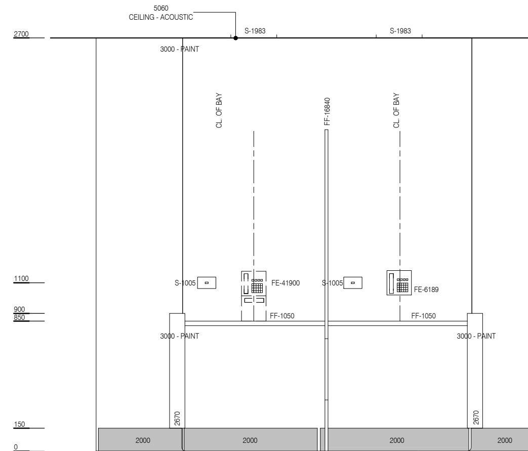
ELEVATION 2
