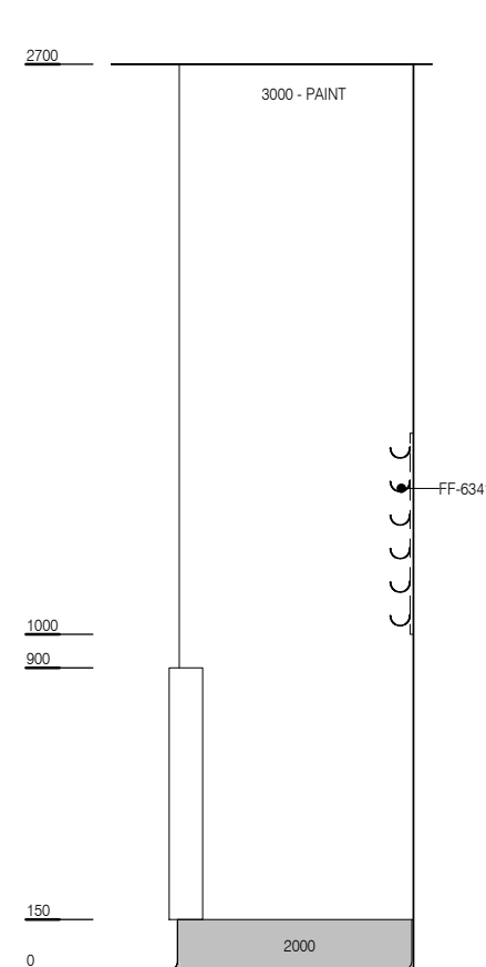
ELEVATION 1
