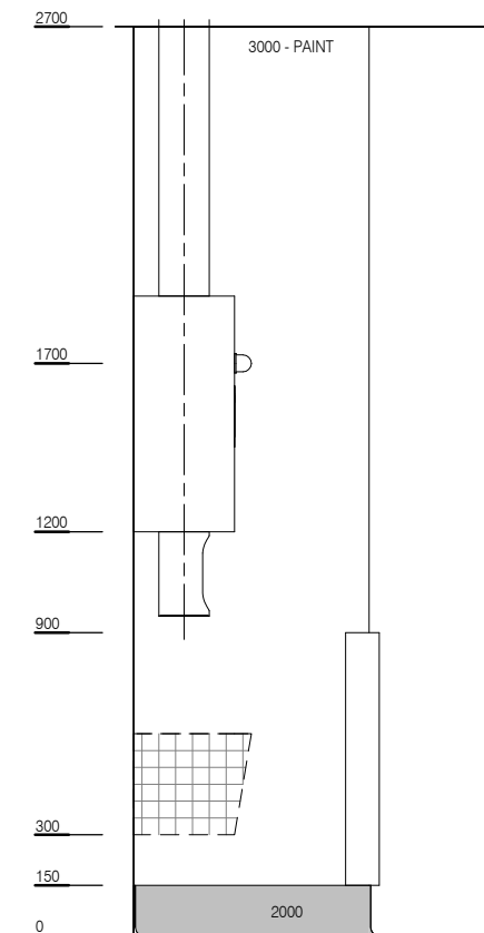
ELEVATION 3
