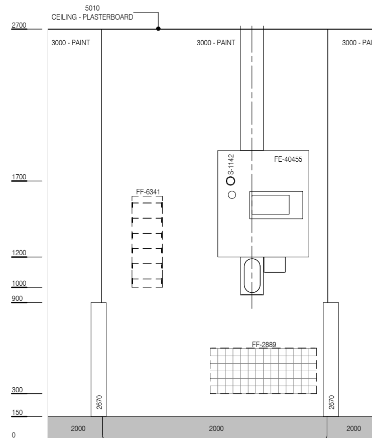
ELEVATION 2
