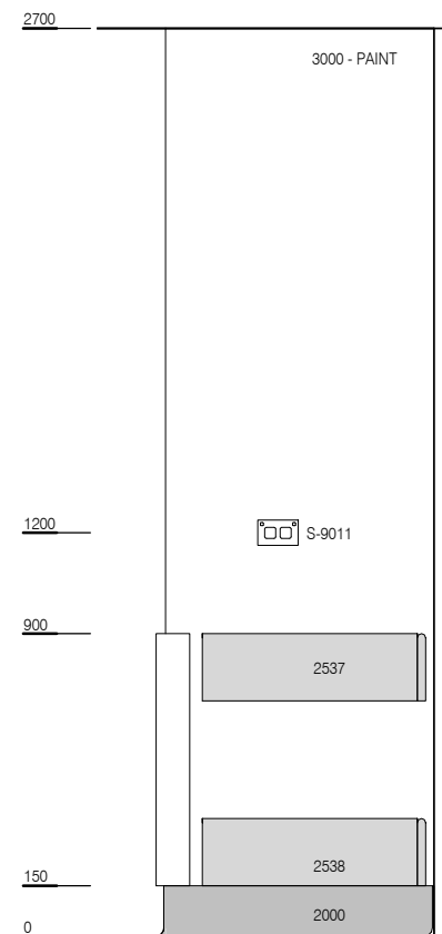
ELEVATION 1
