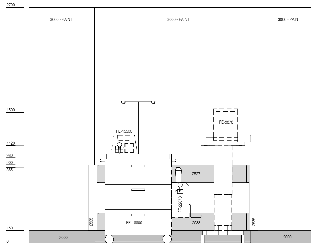
ELEVATION 2
