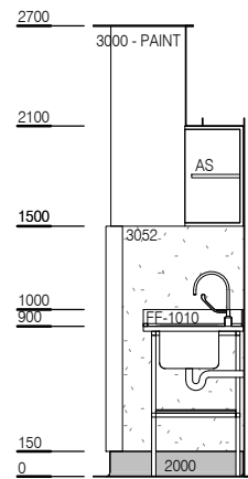
ELEVATION 1
