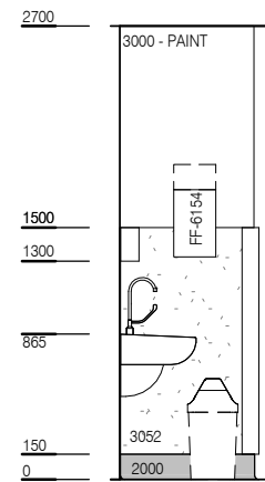
ELEVATION 3
