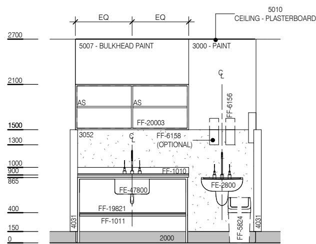
ELEVATION 2
