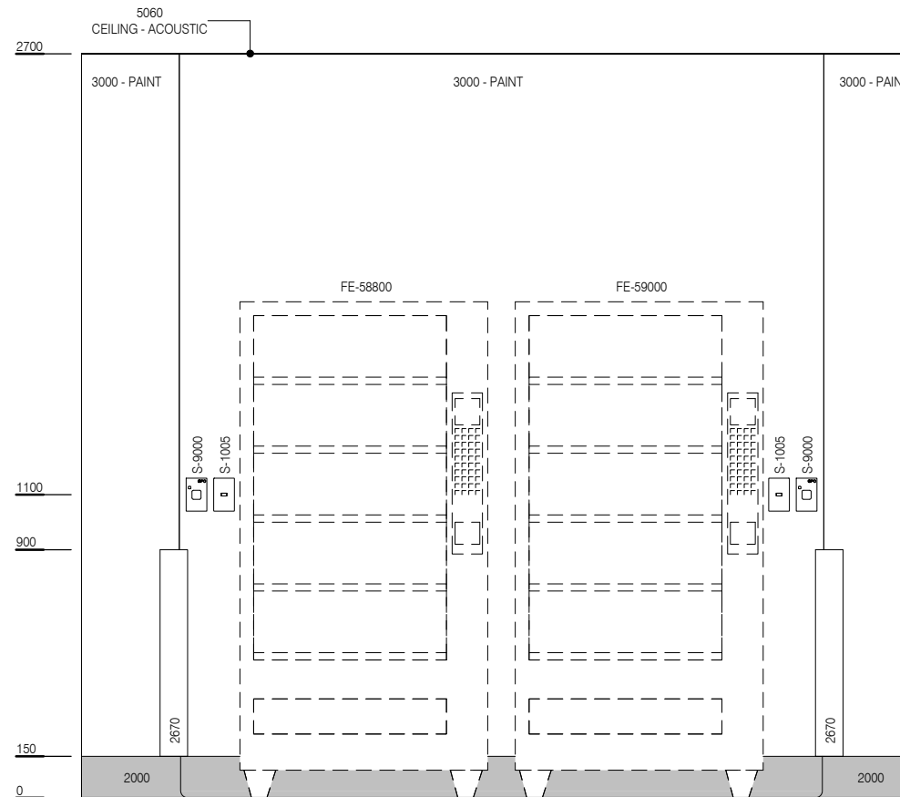
ELEVATION 2
