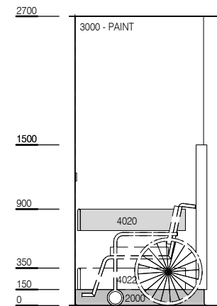
ELEVATION 3
