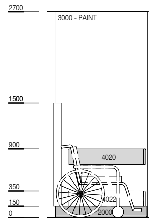
ELEVATION 1
