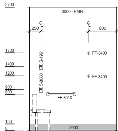
ELEVATION 1
