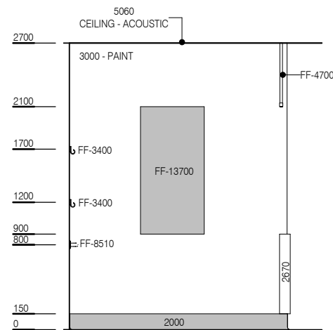
ELEVATION 2
