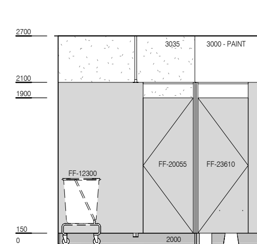
ELEVATION 5
