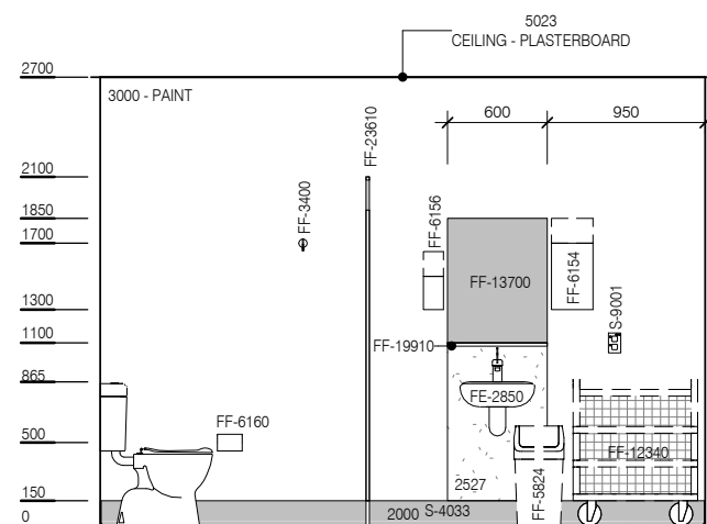
ELEVATION 2
