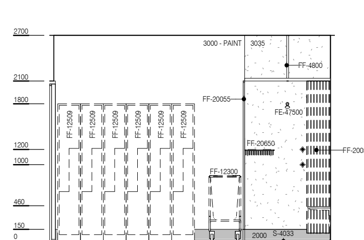
ELEVATION 4
