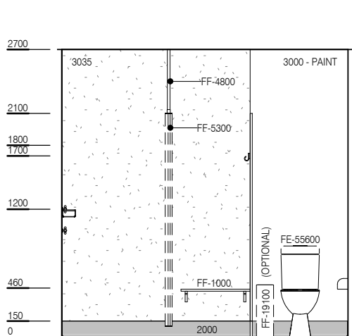
ELEVATION 1
