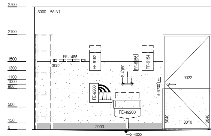
ELEVATION 3
