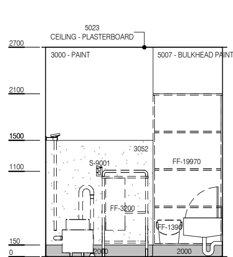
ELEVATION 1
